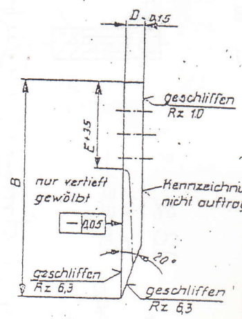
Ansicht Y
