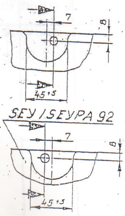
Einzelheit Z
